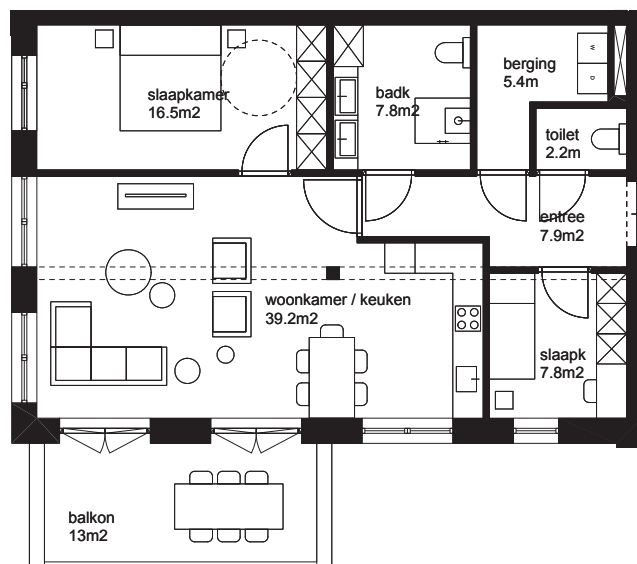
⌚ PLATTEGROND | 1:150
