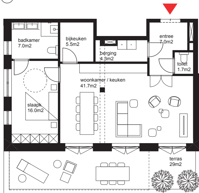
PLATTEGROND | 1:150
